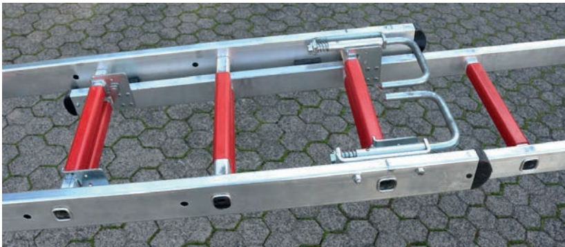
Abbildung 35: Arretiertes Aufsteckteil
