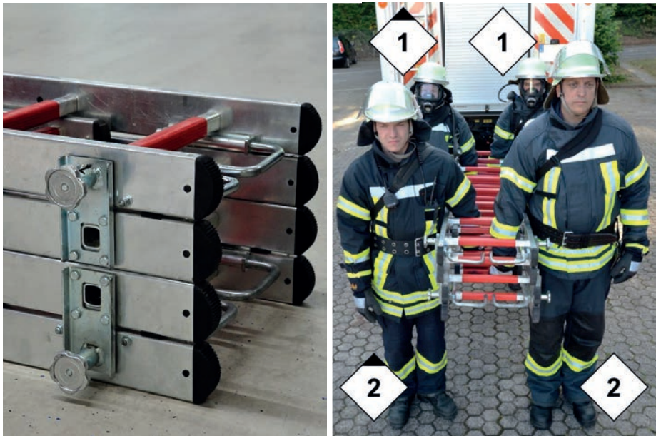
Abbildung 37: Trageweise der Multifunktionsleitern zur Anleiterstelle
