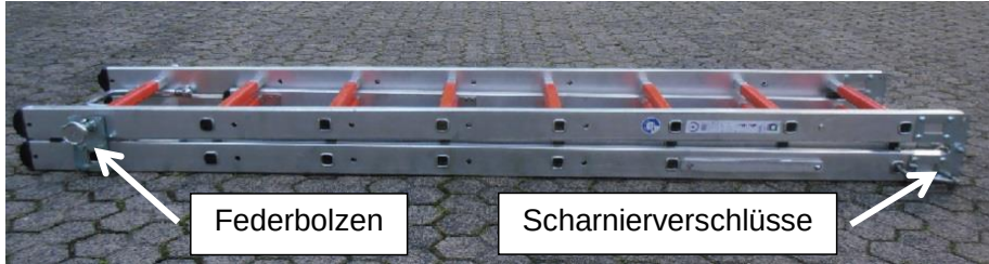
Abbildung 29: Multifunktionsleiter
