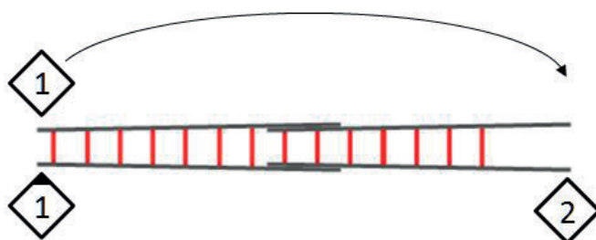
Abbildung 5: Positionswechsel vor dem Zusammenstecken der Steckleiterteile
