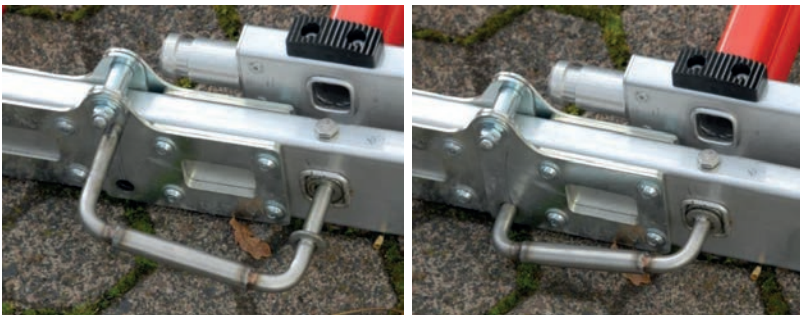
Abbildung 33: Arretieren der Scharnierverschlüsse
