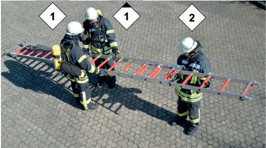
Abbildung 34: Aufstecken des Aufsteckteils
