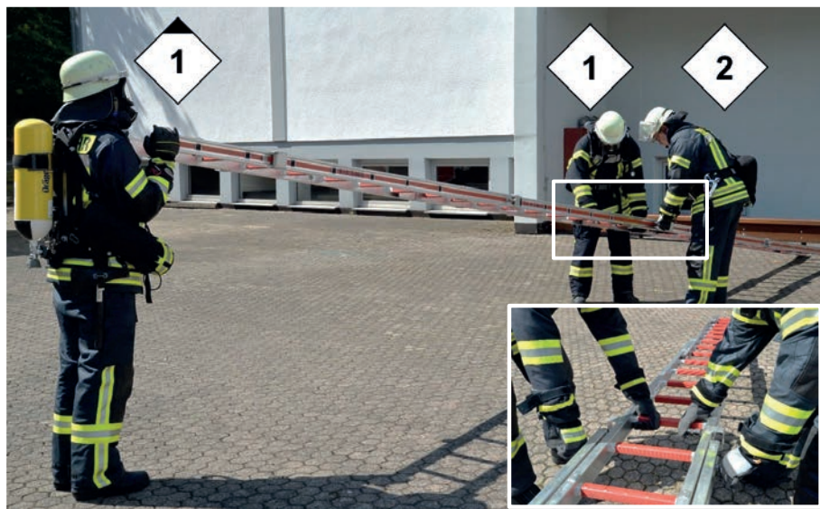
Abbildung 6: Zusammenstecken der Steckleiterteile
